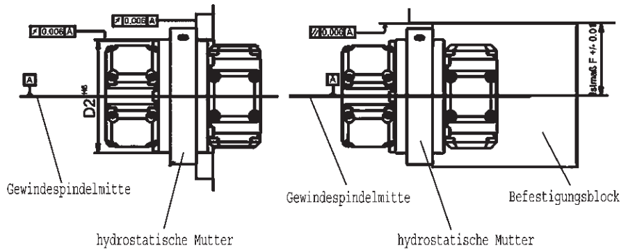
Toleranz bei Flanschausführung
